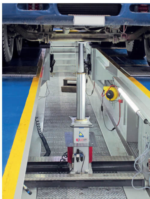
Bild links: Grubenheber Pitlift mit Gelenkspieltester Altus Bild oben: Fertigstahlgrube Rolltec Bild rechts: Absauganlage s.tec
