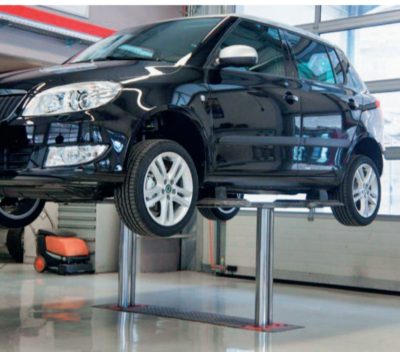
2-Stempel-Bühne Slift Unterflur
