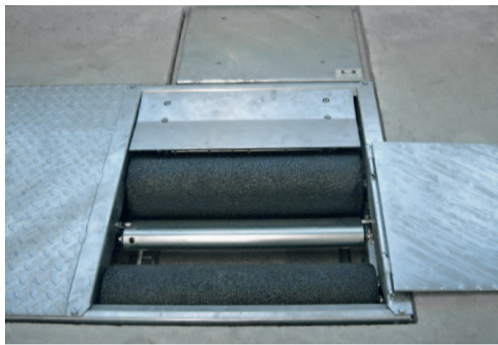
Rollenbremsprüfstand Altus
